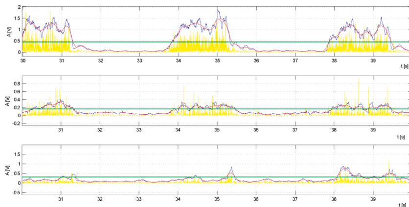
Rysunek 3. Przykładowy przebieg sygnału EMG na trzech kanałach nagrany z powierzchni skóry barku w trakcie skokowego przemieszczenia kończyny górnej
