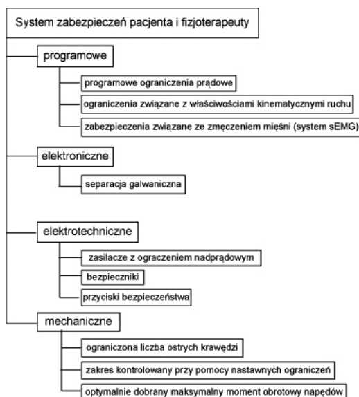
Rysunek 6. System zabezpieczeń robota ARR
